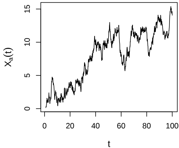
c=8
