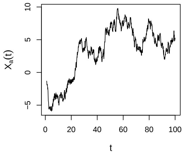
c=2
