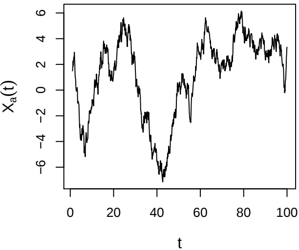
c=5
