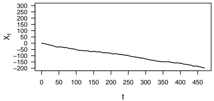
p = 0.3 q = 0.7 r = 0
