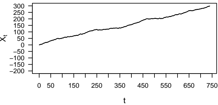
p = 0.7 q = 0.3 r = 0
