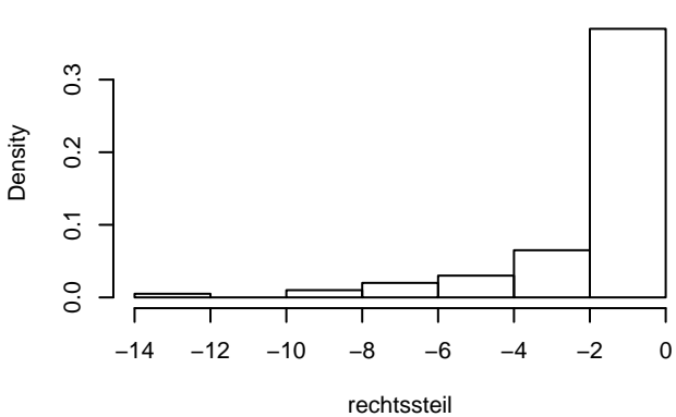
Rechtssteile Verteilung
