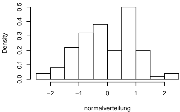
Normalverteilung
