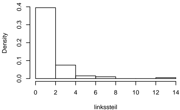
Linkssteile Verteilung
