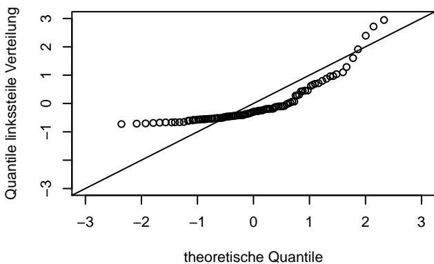
Normal-Q-Q-Plot
