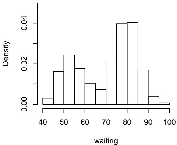
Histogramm: Standardeinstellung
