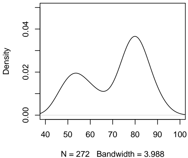
Kerndichtschätzung: Standardbandweite
