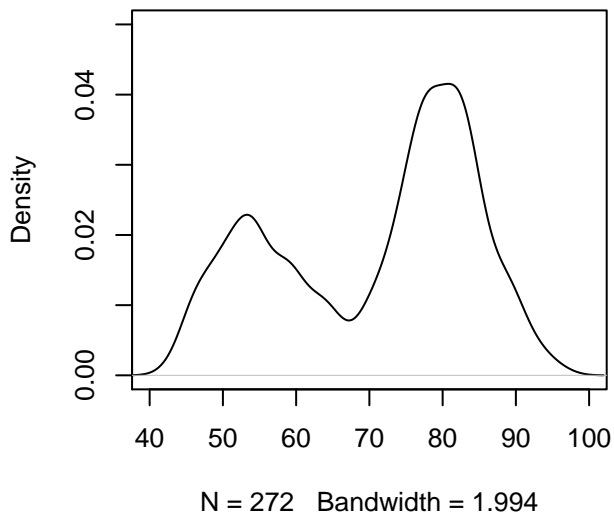
Kerndichtschätzung: 'adjust = 0.5'
