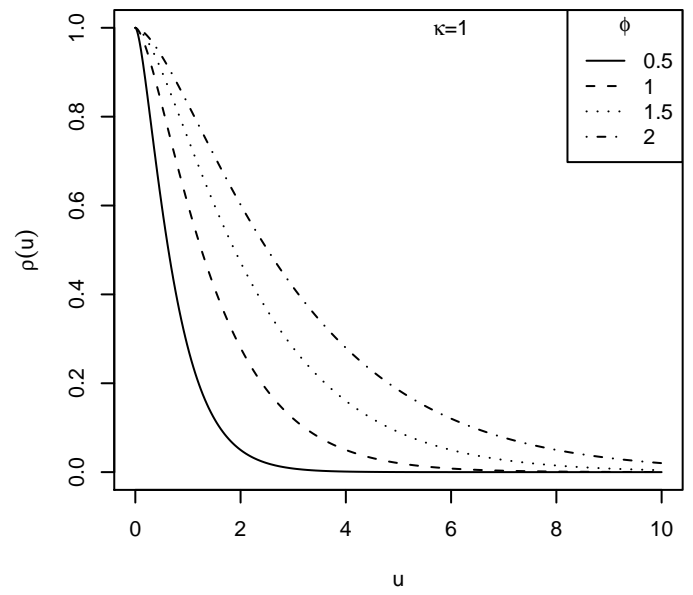
Matern-Familie
