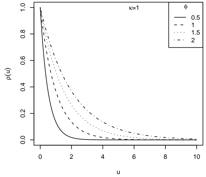
Potenz-Exponentialfamilie
